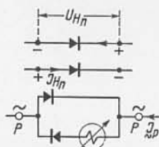
Bild 6. Halbwellenschaltung.
