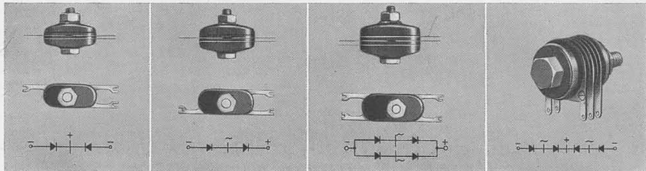
Bild 1 bis 3. Meßgleichrichter in Preßstoffgehäuse. 1 mA Form G 1321/1
