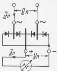
Bild 5. Graetzschaltung.
